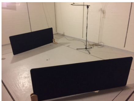
Fig. 1: Mätuppställning ScreenIT A30 1800 x 650 mm
